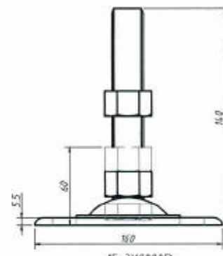
15-3Y2000B 水平調整 70mm 2t タイプ
