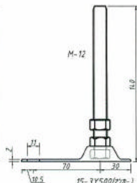
15-3Y500(ﾌﾟﾗﾝ-) 水平調整 85mm 500kタイプ
