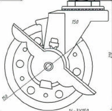
14-3Y150 160K ストッパー付タイプ
