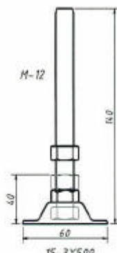
15-3Y500 水平調整 85mm 500kタイプ
