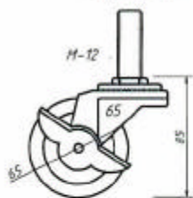
14-3Y65 30K ストッパー付タイプ
