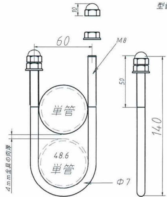
安全化粧キャップ×2 セムスナット×2 型番-28-2U-140
