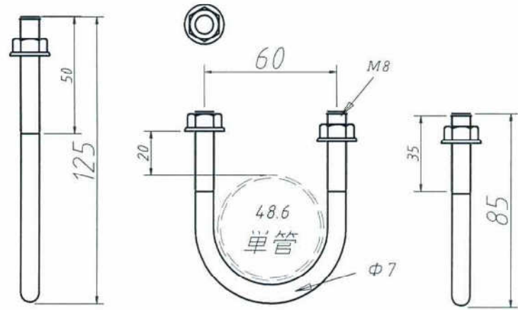
セムスナット×2 型番-28-1U-85
