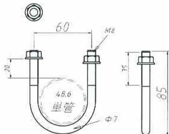
セムスナット×2 型番-28-1U-85
