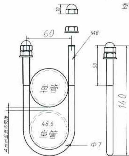
安全化粧キャップ×2 セムスナット×2 型番-28-2U-140
