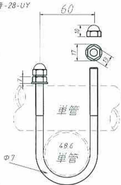
安全化粧キャップ×2 セムスナット×2 型番-28-2U-125
