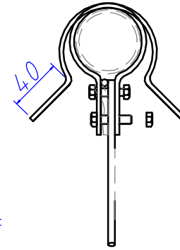
FIT-KK カシメ金具
