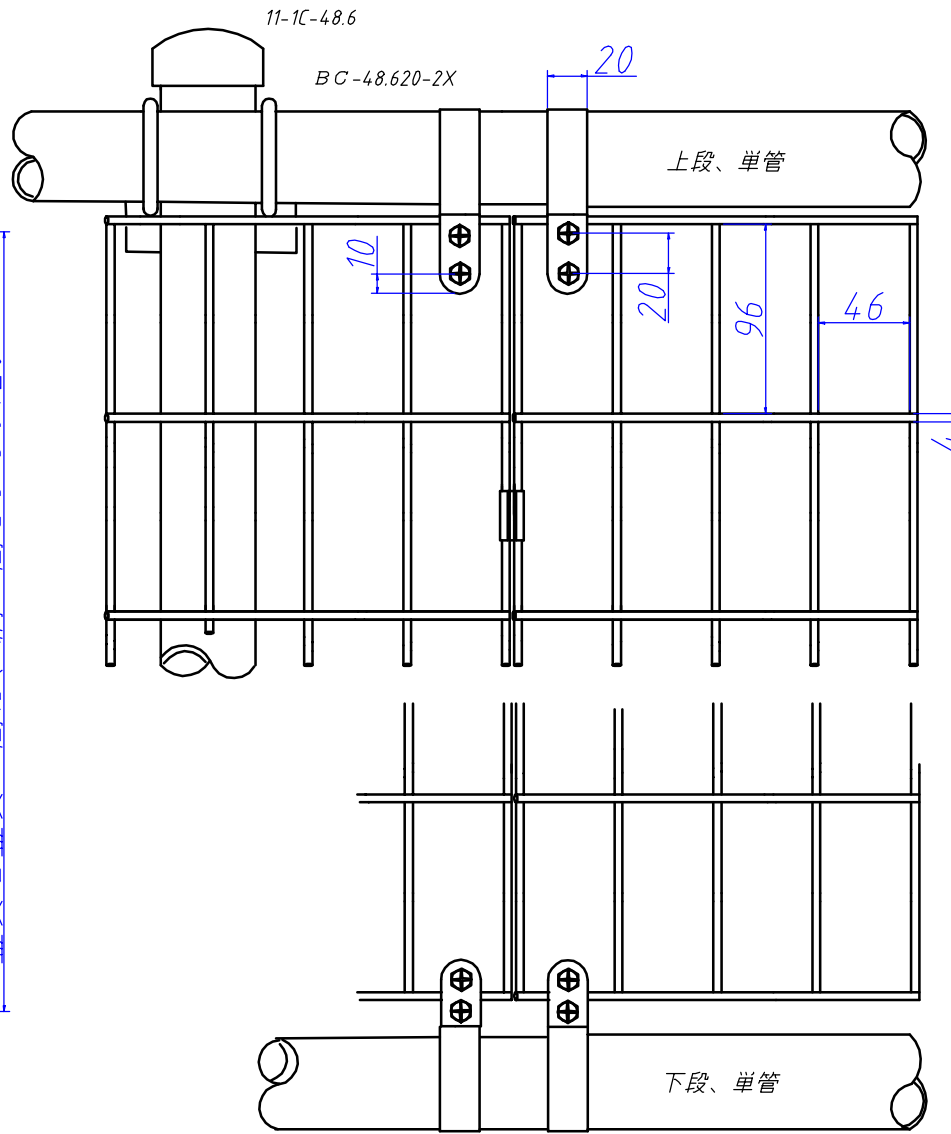
FIT-FK 取付金具
