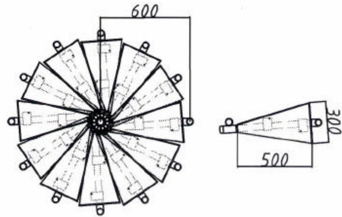
R-CPL 階段プレート (2.3t)
