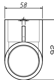
15-2L500 タテ
