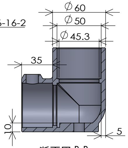
断面図 P-P スケール 1 : 2.5
