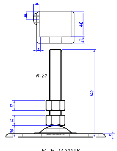
S-15-1A2000B 水平調整70mm 2t タイプ
