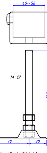
S-15-1A500A(アンカー) 水平調整85mm 500tタイプ
