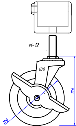
S-14-1C100 50Kストッパー付タイプ
