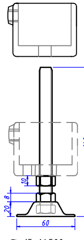
S-15-1A500 水平調整85mm 500tタイプ
