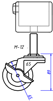
S-14-1C65 30Kストッパー付タイプ
