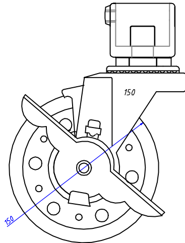
S-14-1C150 160Kストッパー付タイプ
