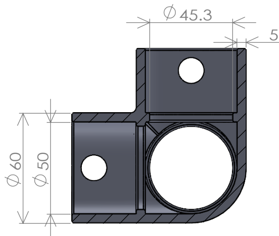
断面図 A-A
