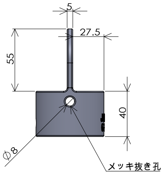
断面図 A-A
