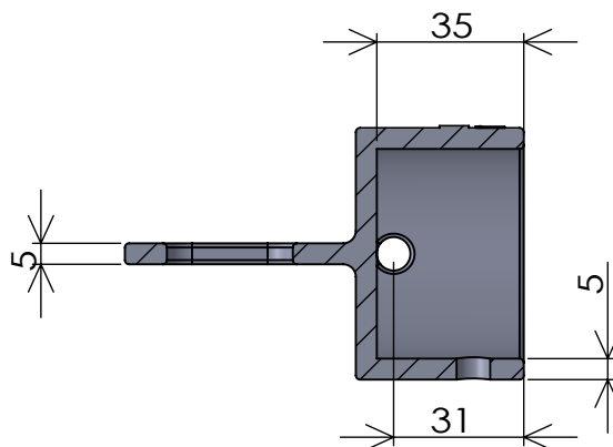
断面図 A-A
