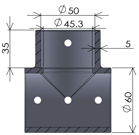
断面図 Q-Q
