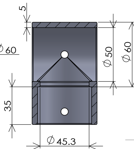
断面図 A-A
