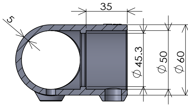
断面図 A-A
